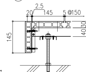
② 端部部納まり図 (S=1/10)
