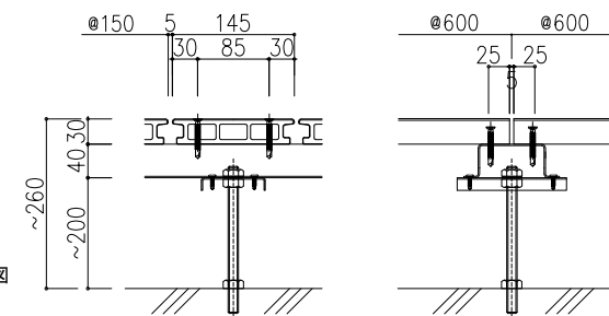
① 標準部納まり図 (S=1/10)
