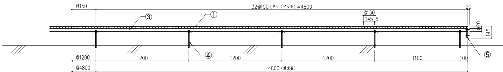
断面図 (S=1/30)
