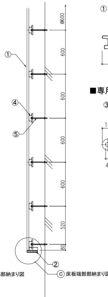
断面図 (S=1/30)
