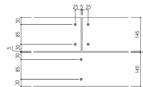
④ ビス固定位置図 (S=1/10)
