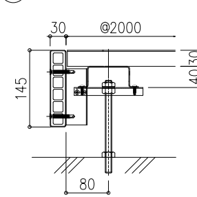
③ 床板端部部納まり図 (S=1/10)
