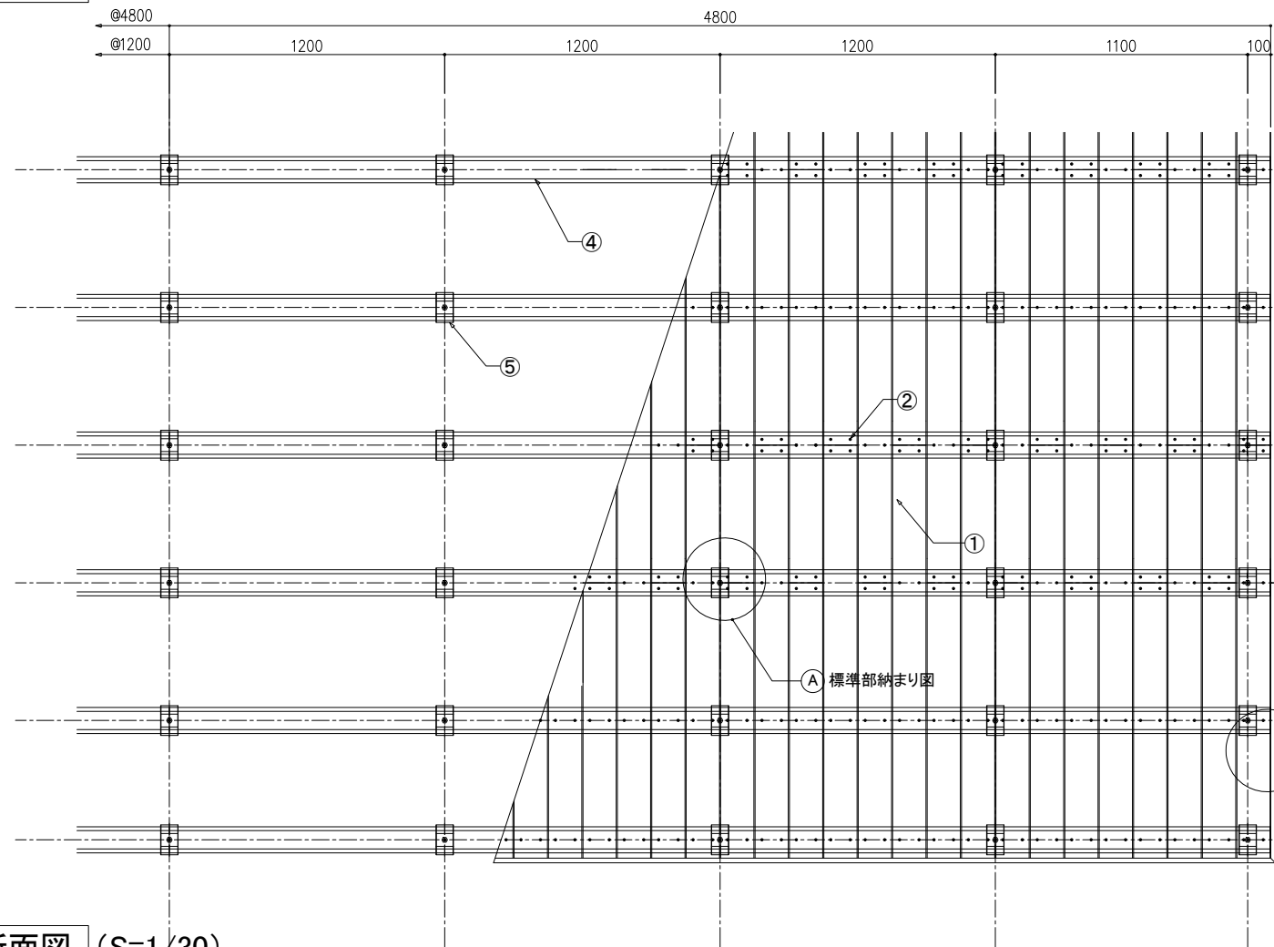
平面図 (S=1/30)
